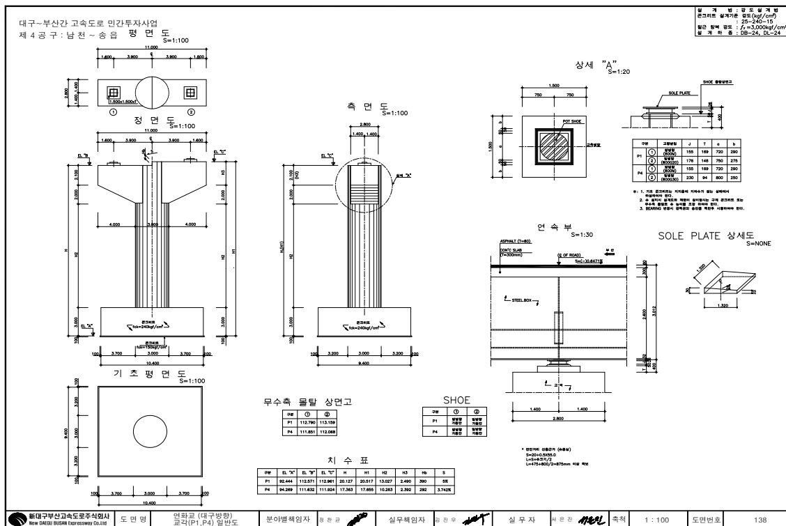
<교각 일반도>
