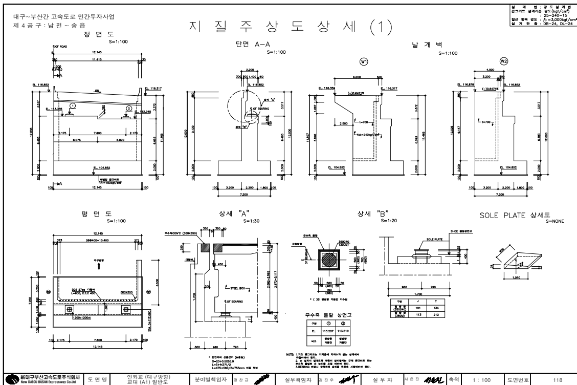
<교대 일반도>
