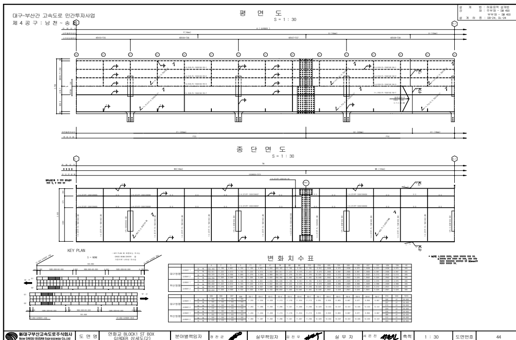
〈강상형 상세도〉
