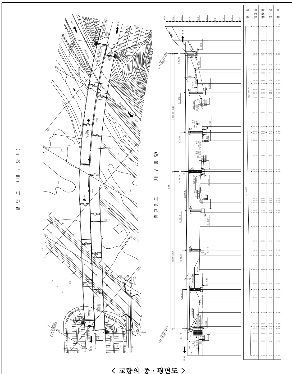
【그림 1.4.1】 삼성1교(대구) 종·평면도
